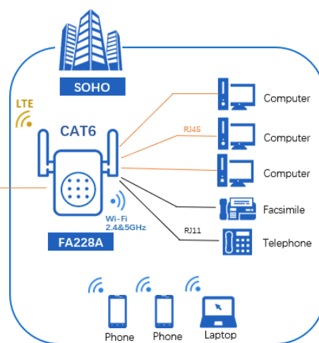
Scenario2-SOHO FA228A
